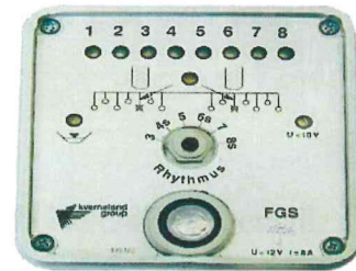
Kontrolní a ovladačí panel FGS elektroniky pro jednoduchou a přehlednou práci
