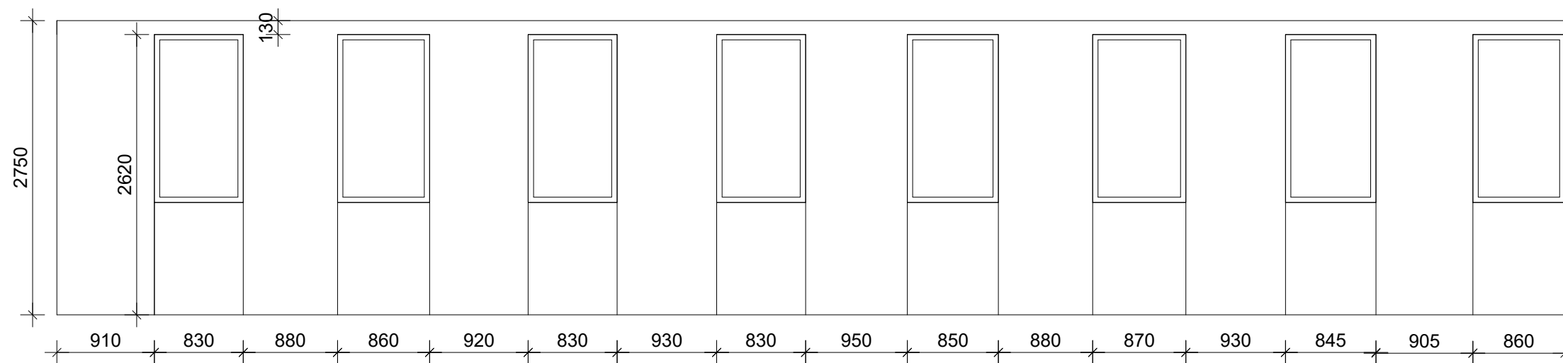
ROZVINUTÝ POHLED
