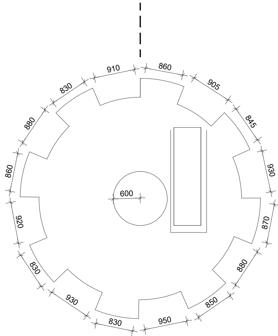
PŮDORYS
