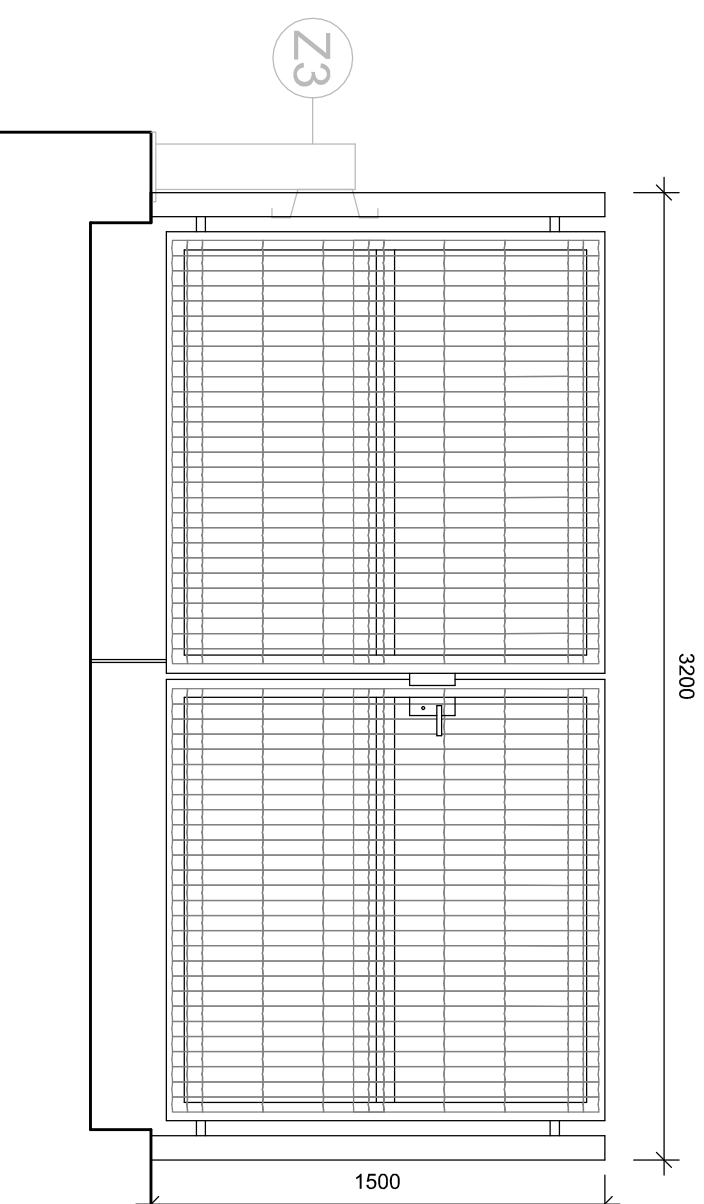
POHLED NA DVOUKŘÍDLLOU VJEZDOVOU BRÁNU DVOUKŘÍDLA VJEZDOVA BRÁNA Z1
