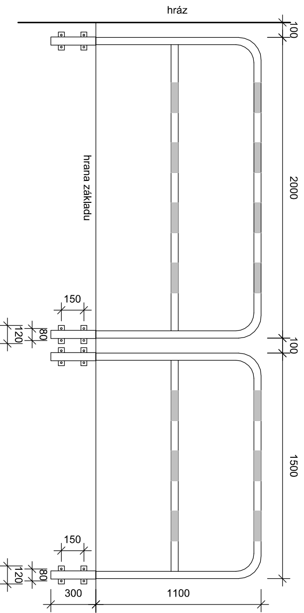
POHLED Z ČELA NA HRANU ZÁKLADU (SJEZDU) ODNIMATELNÉ ZÁBRADLÍ Z4
