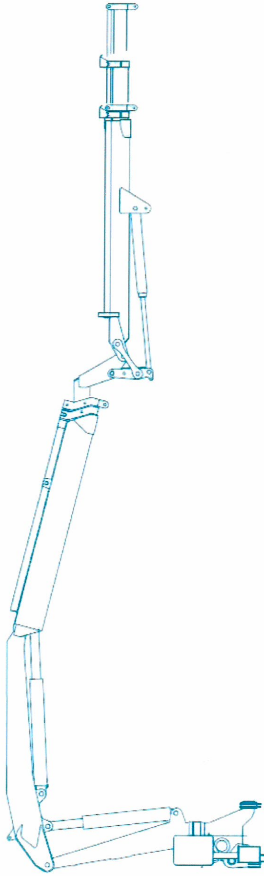
Jeřáb s přídavným ramenem
