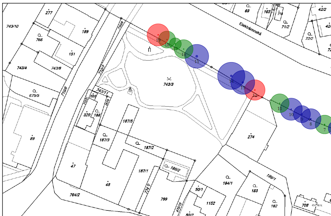
Krčín, ř. km 16,700 - 17,900(1:700), 9/10
