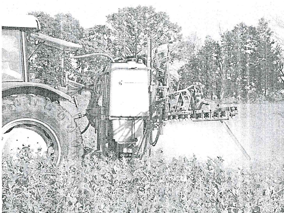
Foto postřikovače UNIA LUX 812:
