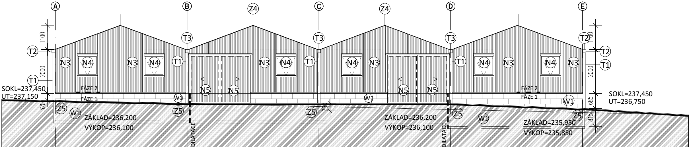
POHLED JIŽNÍ
