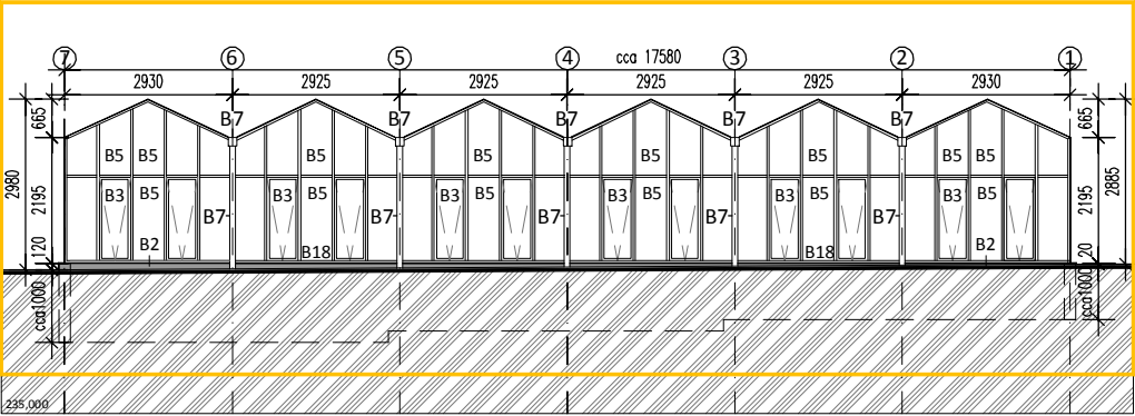
POHLED SEVERNÍ
