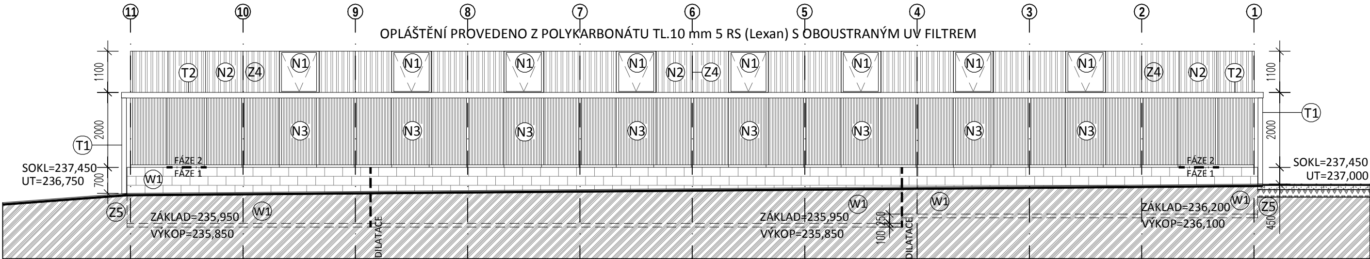
POHLED VÝCHODNÍ
