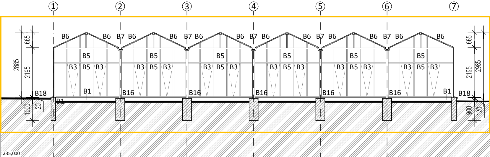
ŘEZ A-A
