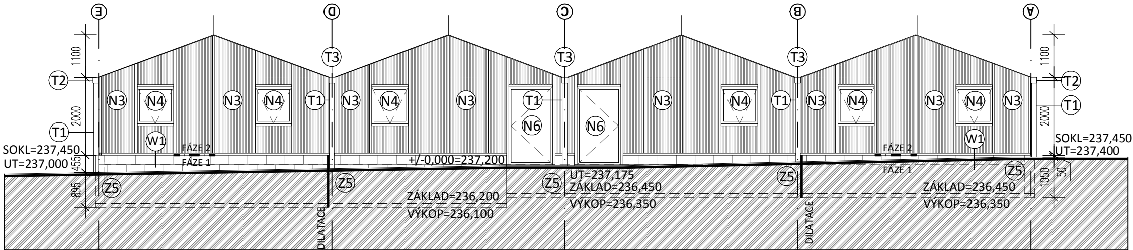
POHLED SEVERNÍ
