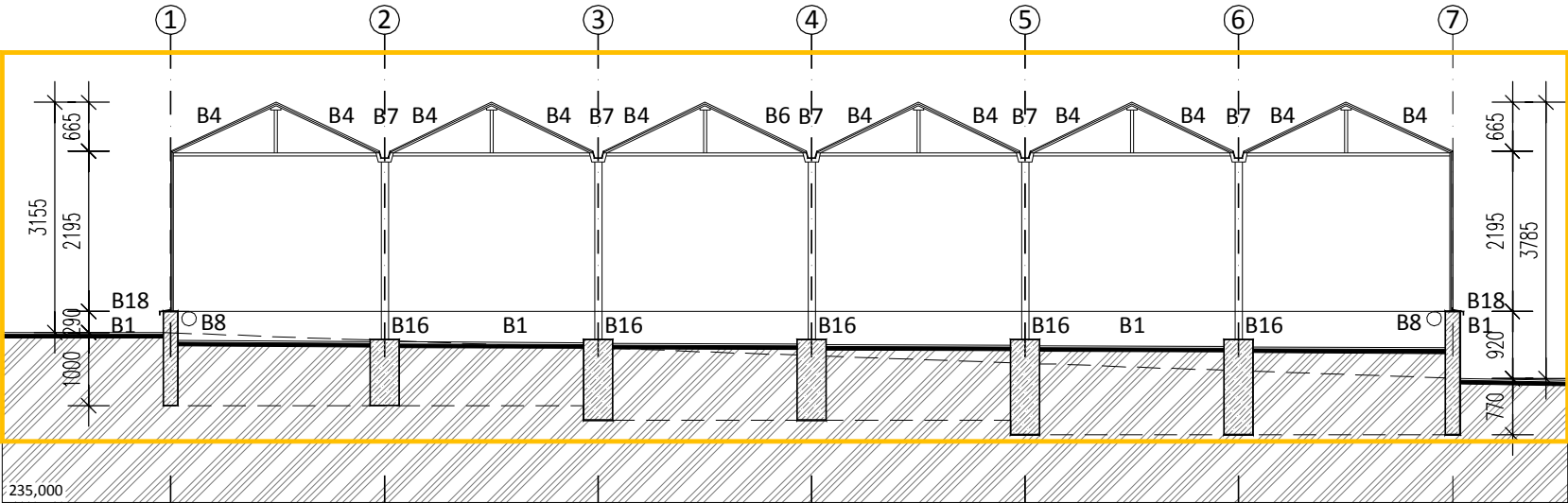
ŘEZ B-B
