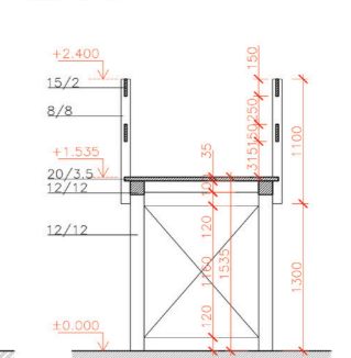
Řez B-B'
