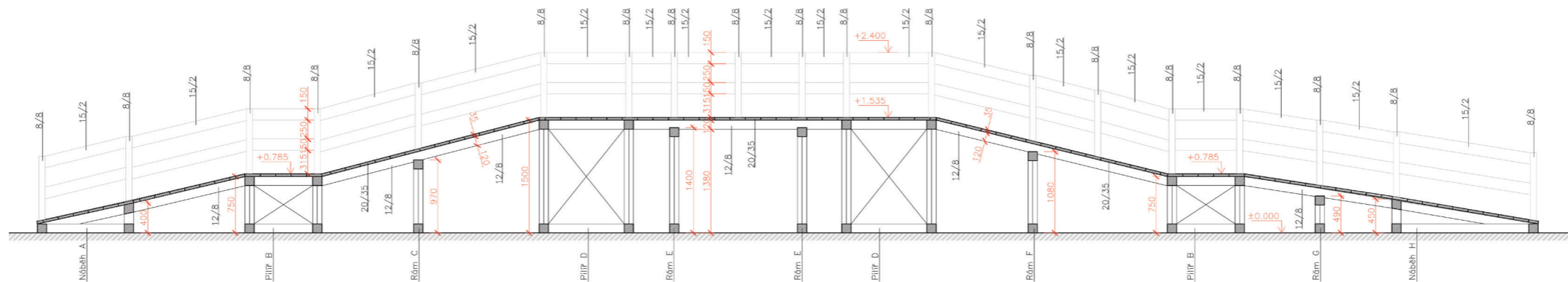
Rozvinutý řez A-A'
