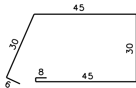
① 1 ø 6 á 25cm, dl 162 cm
